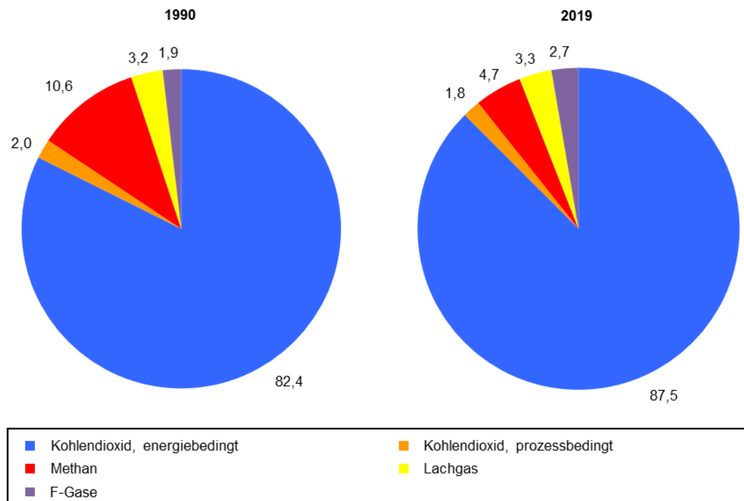
Abbildung 17 Struktur der Gesamtemissionen in Hessen in CO 2 -Äquivalenten in den Jahren 1990 und 2019
